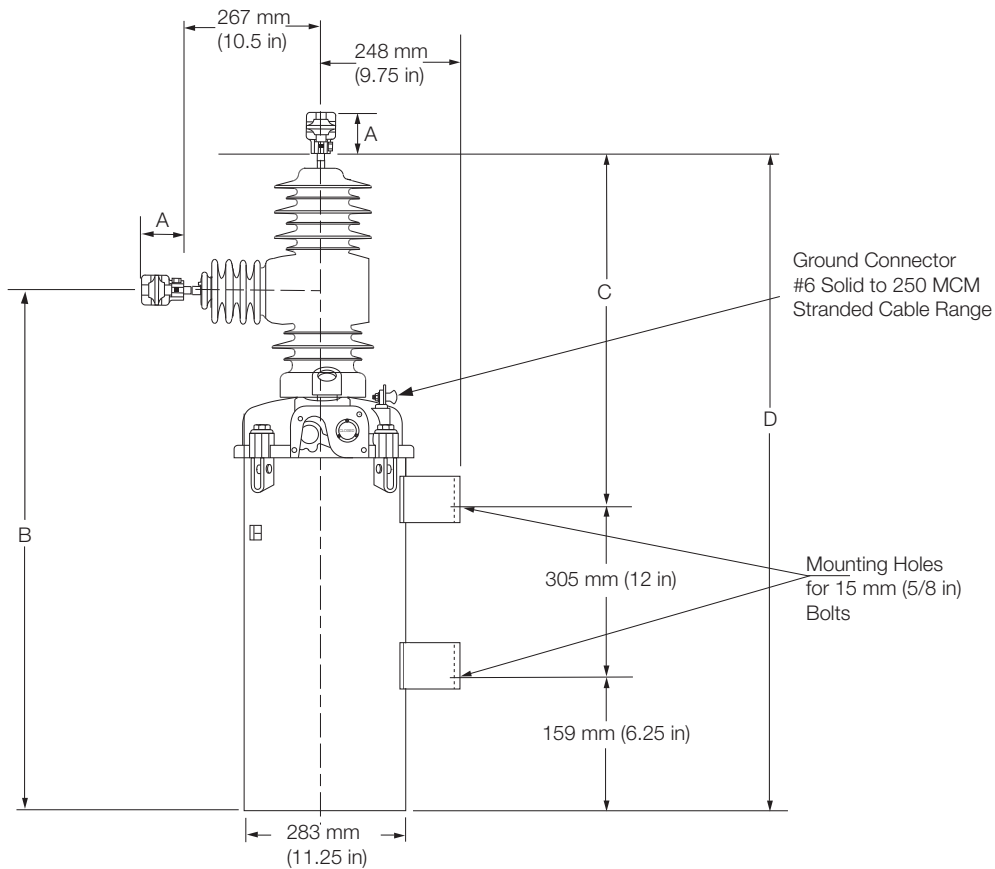
NOVA-TS Dimensions
